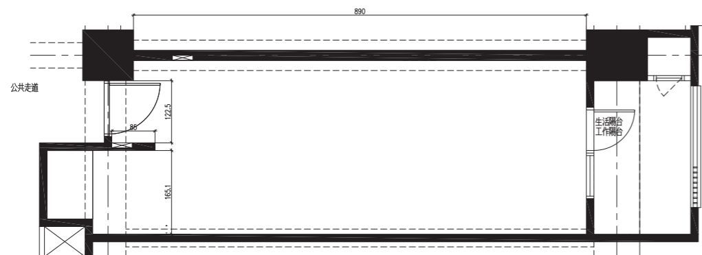
一房型TYPE-A住宅單元平面圖 比例：A3:1/100 A1:1/50
