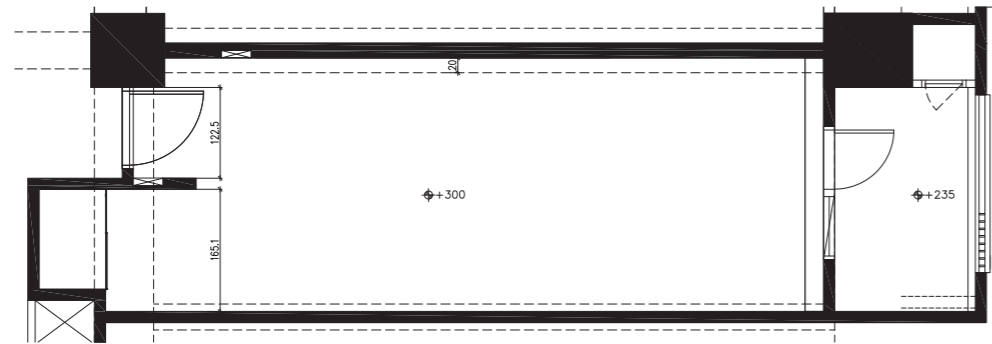
一房型TYPE-A住宅單元天花平面圖 比例：A3:1/100 A1:1/50
