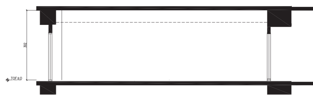
一房型TYPE-A住宅單元剖立面圖 比例：A3:1/100 A1:1/50
